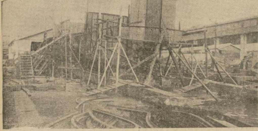
Tersanemizde hali inşaada ovr gemi teknesi
